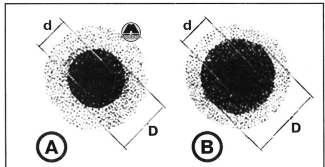
A) Масло с низким уровнем диспергирующих свойств, B) масло с высоким уровнем диспергирующих свойств.
