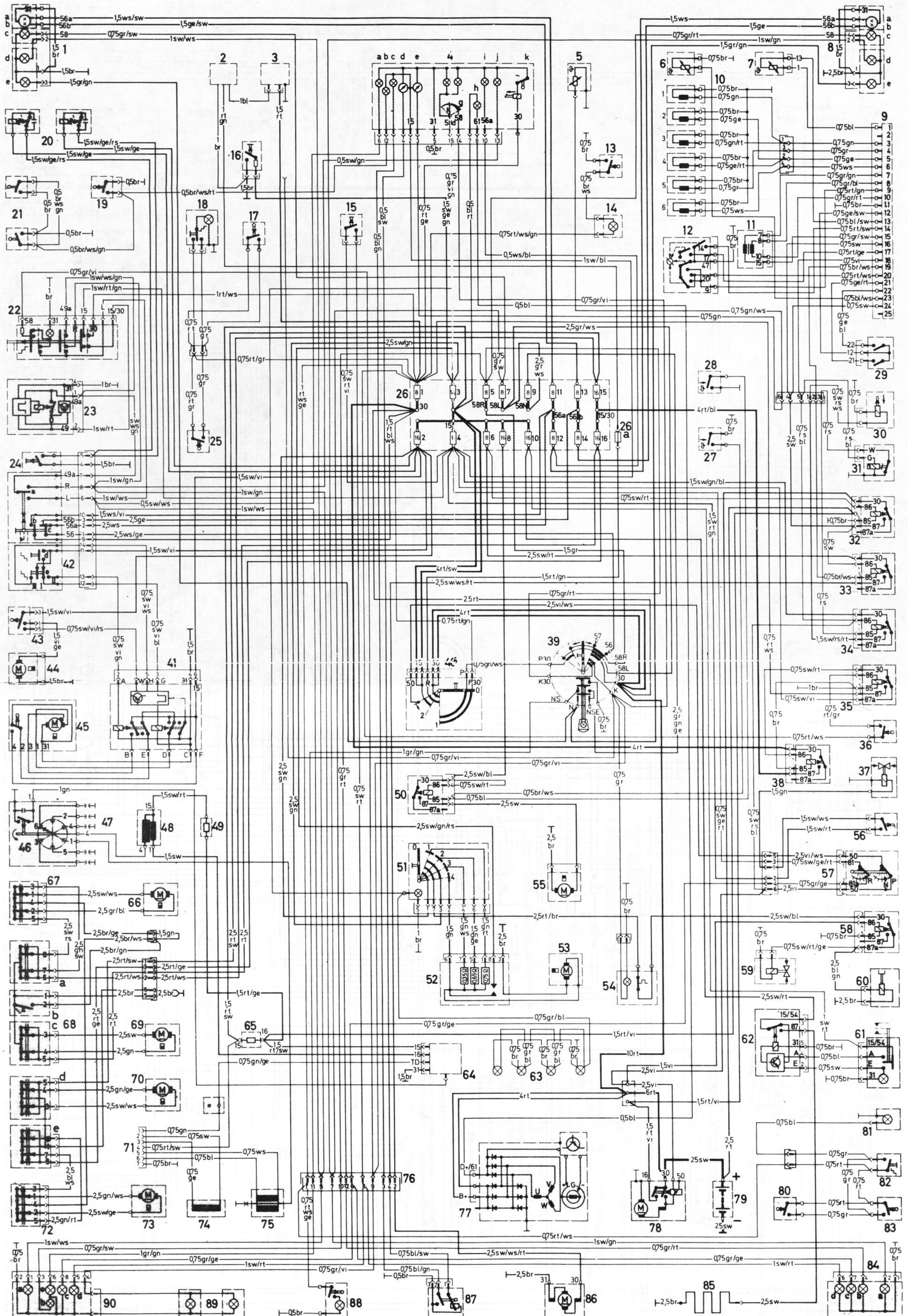
Схема электрооборудования 280 SE
