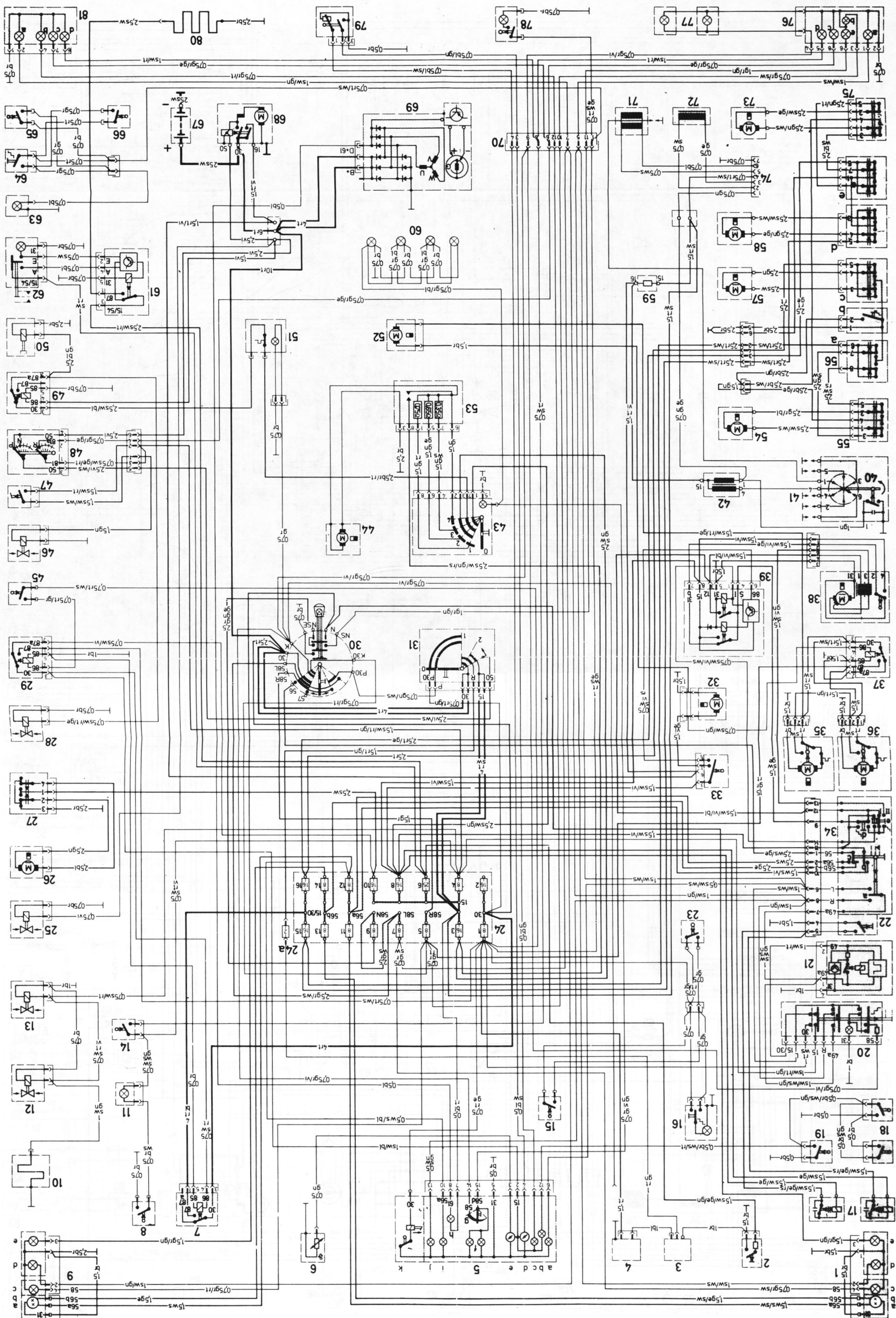
Схема электрооборудования 280 S
