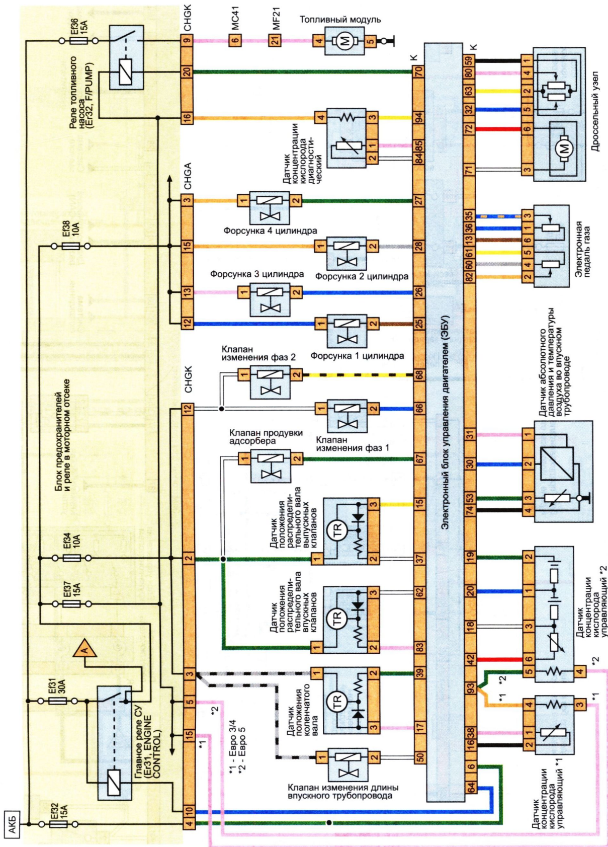
Схема 1.1. Система управления двигателем
